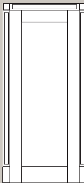
OPASKI OZDOBNE OP-2 KOSTKI GÓRNE SŁUPKI DOLNE (PRZYKŁAD MODEL FZ-0) Opcja za dopłatą
