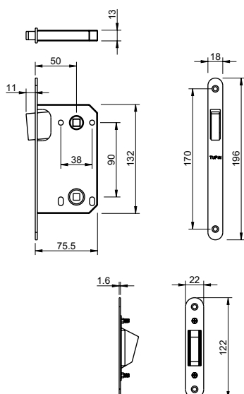
Fechadura magnética WC WC 6 mm Quadrado de 8 mm
