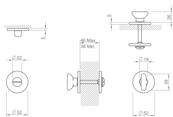
Conjunto de Botão WC Adaptador metálico Ferro quadrado 4,6,8 mm
