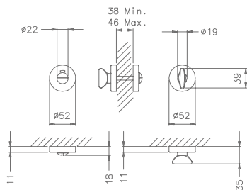
Conjunto de Botão WC Adaptador metálico Ferro quadrado 4,6,8 mm
