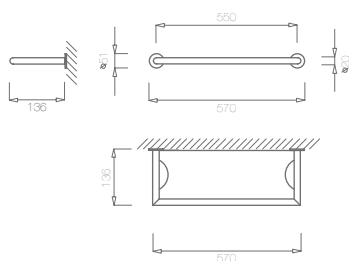
Prateleira de vidro 570mm de comprimento Roseta de Ø51mm Sistema de fixação invisível
