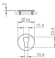
Espelho chave par Entrada cilindro europeu
