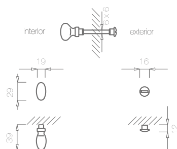
Conjunto para WC com botão oval fêmea Ferro quadrado simples 6x60mm
