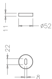
Espelho chave par Adaptador metálico ou plástico
