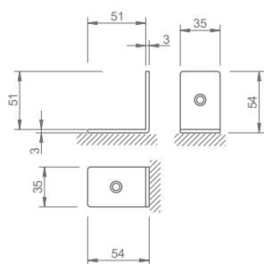
Parede/placa Suporte para painel Aparafusa de um lado os painéis Fixa do outro lado à parede 1 bucha plástica, 1 parafuso, 1 porca especial e 1 parafuso métrico
