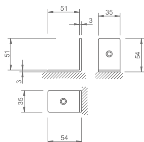
Placa/placa Suporte para painel Aparafusa de um lado os painéis Fixa do outro lado à parede 2 porcas especiais e dois parafusos métricos
