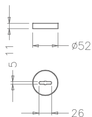
Espelho chave par Adaptador metálico ou plástico
