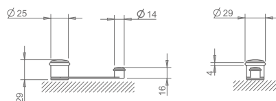
Batente duplo com fixação de porta
