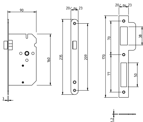
Fechadura passagem 55, 60mm distância da testa à broca Com cantos redondos sob pedido
