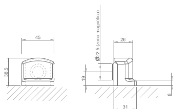
Batente de porta magnético
