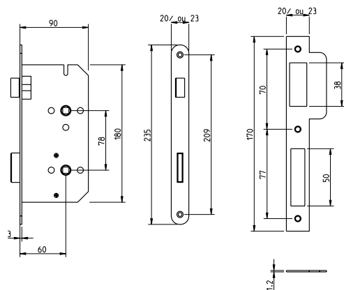
Fechadura WC 55, 60mm distância da testa à broca Com cantos retos sob pedido
