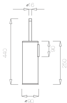
Porta piaçaba de parede Escova e suporte com copo de plástico para protecção interior
