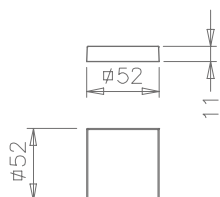
Espelho de chave par oculto Adaptador metálico
