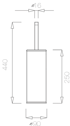
Porta piaçaba de chão Escova e suporte com copo de plástico para protecção interior
