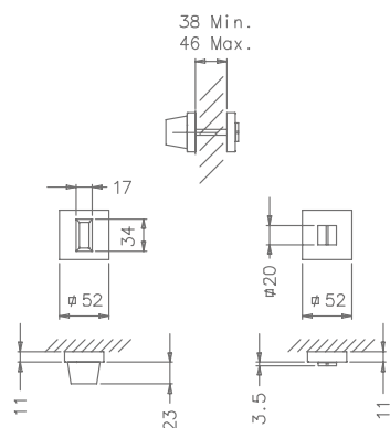
Conjunto de Botão WC Adaptador metálico Ferro quadrado 4,6,8 mm
