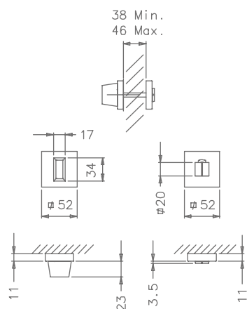
Conjunto de Botão WC Adaptador metálico Ferro quadrado 4,6,8 mm
